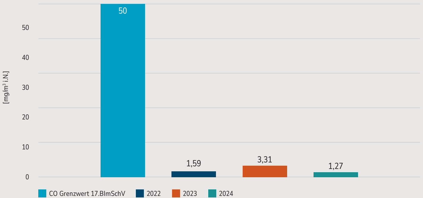
Abbildung 5: Tagesmittelwerte CO
