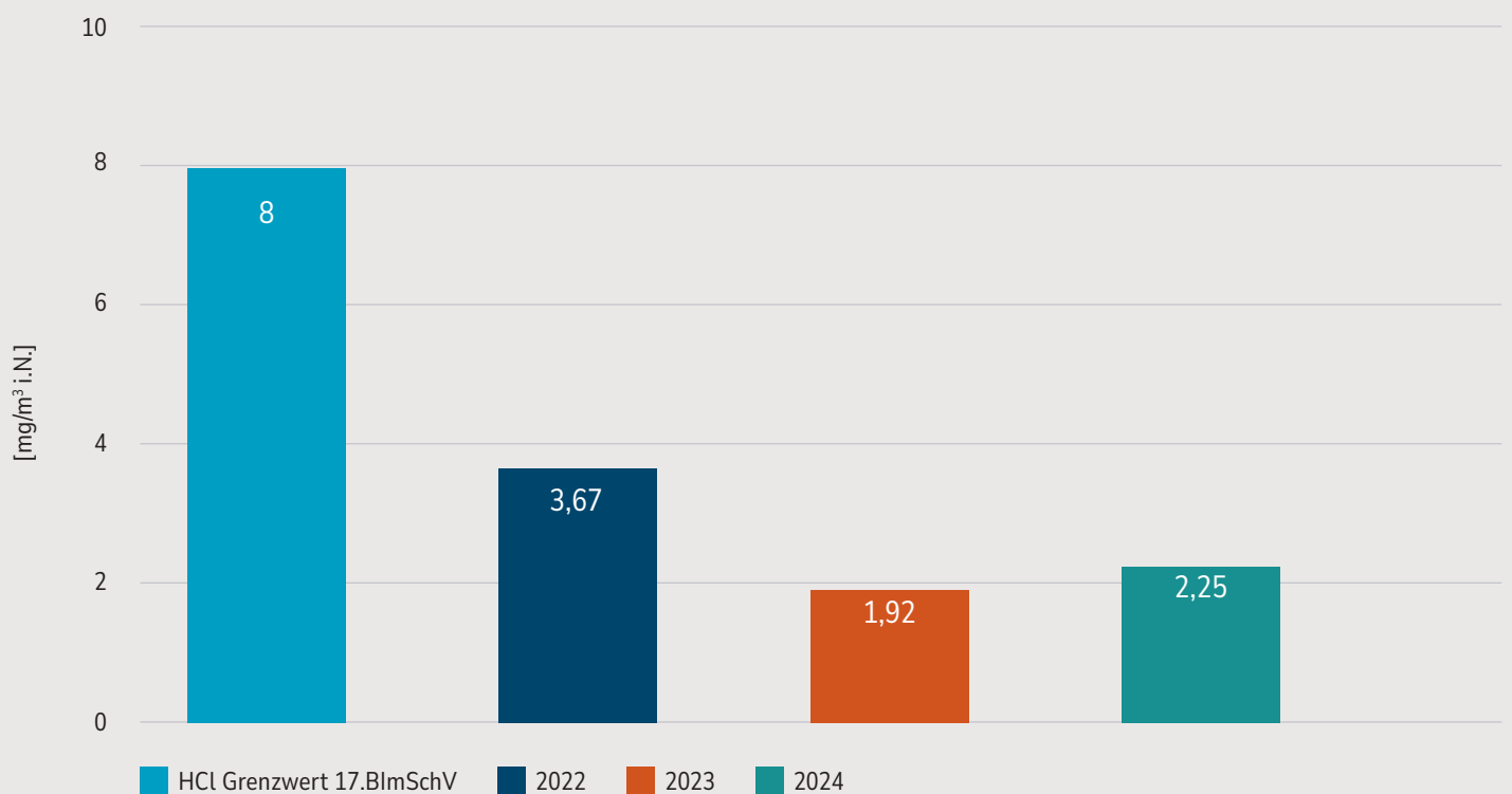
Abbildung 4: Tagesmittelwerte HCl
