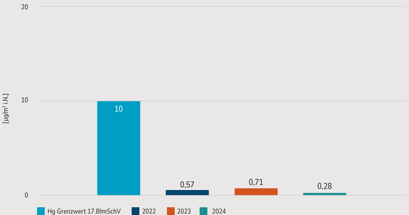
Abbildung 9: Tagesmittelwerte Hg
