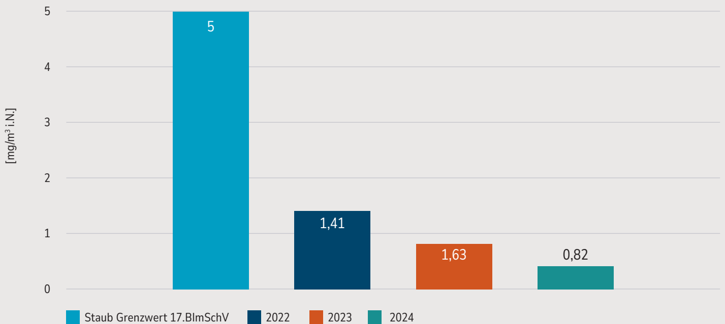
Abbildung 10: Tagesmittelwerte Staub
