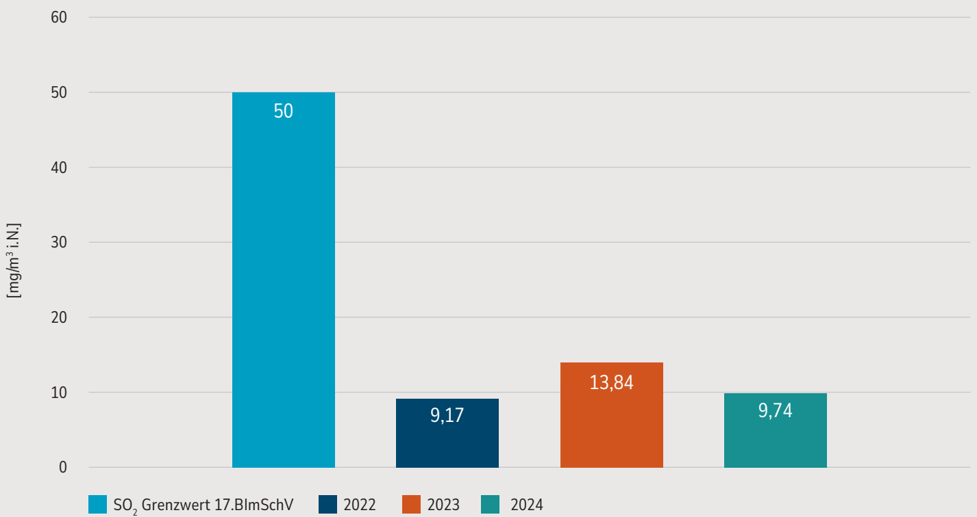
Abbildung 7: Tagesmittelwerte SO 2
