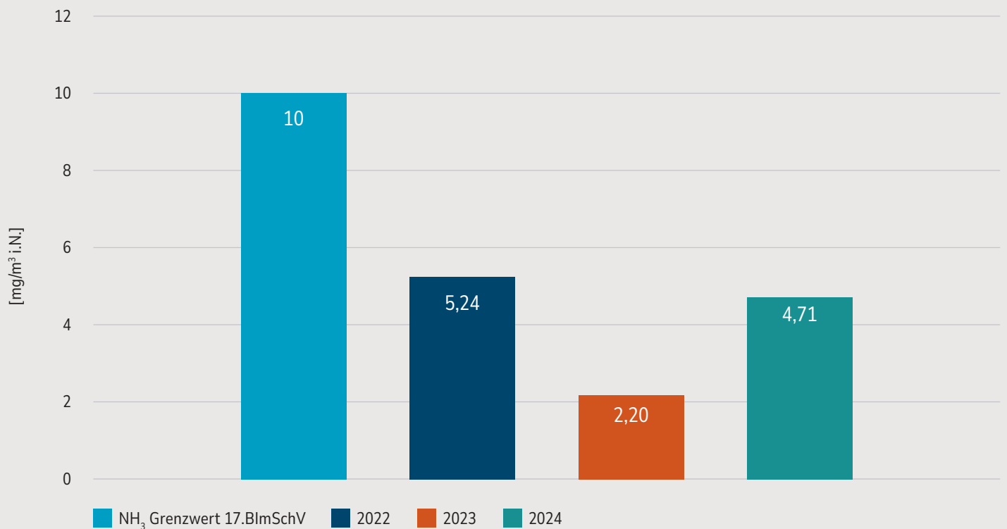
Abbildung 11: Tagesmittelwerte NH 3
